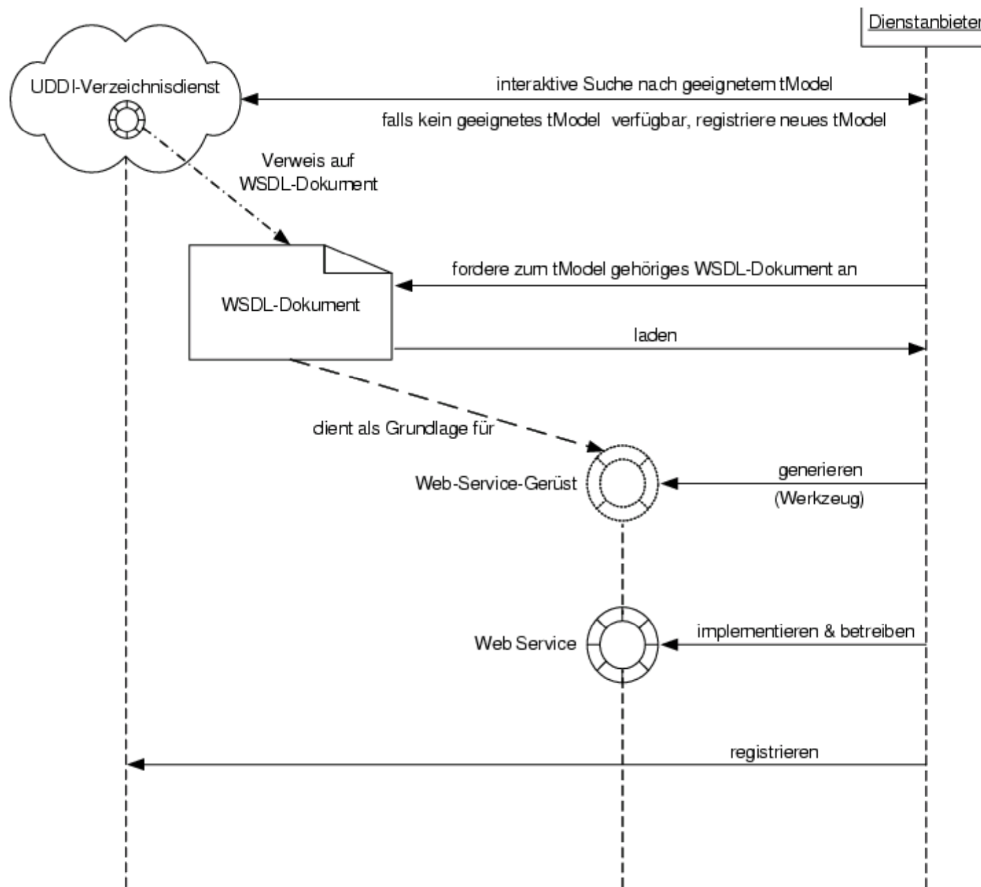
Abb. 19.11: Aktionen zum Erstellen des Web-Services
