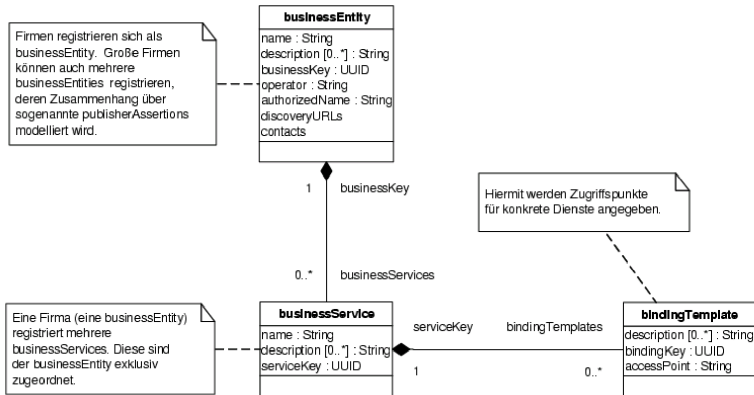
Abb. 19.13: Zusammenhang der UDDI-Komponenten
